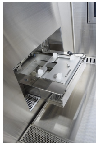
培養容器自動傳遞平台
