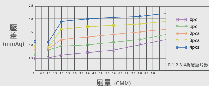
配重性能曲線表
